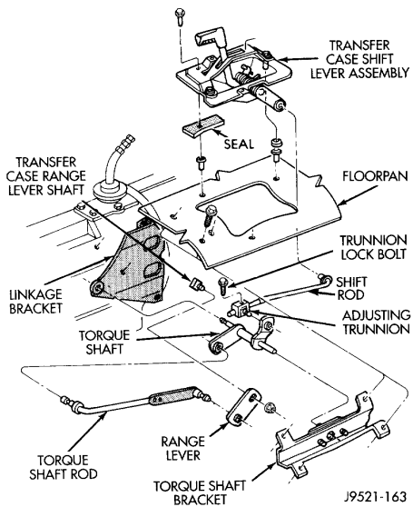
Fig. 87 Shift Linkage
