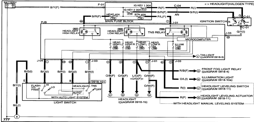
0918-101 LIGHT SWITCH
